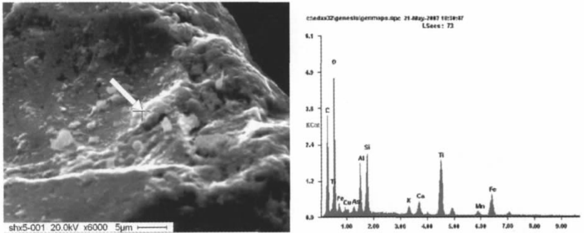
图 4 环境扫描电子显微镜颗粒形貌及 X 射线能谱分析图(箭头指向能谱分析点)
