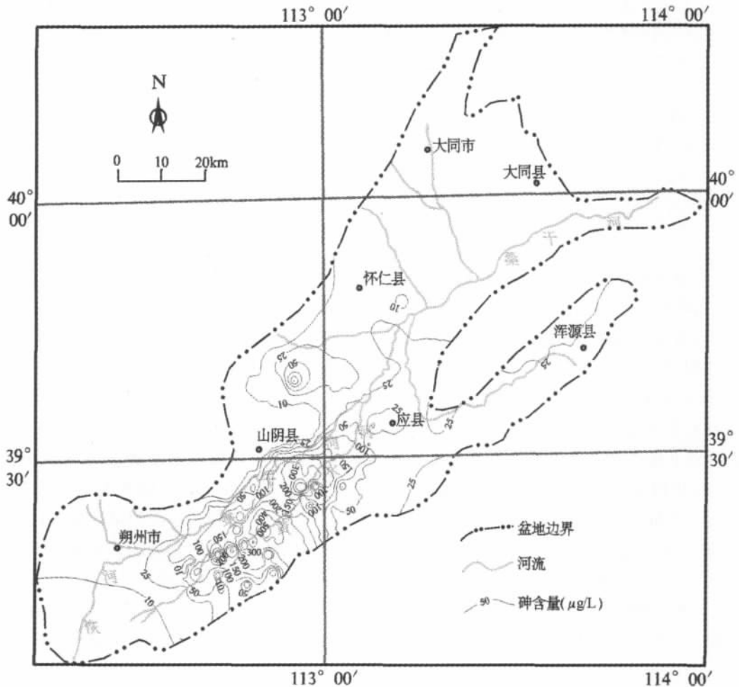
图 1 大同盆地浅层地下水中砷含量等值线分布图
