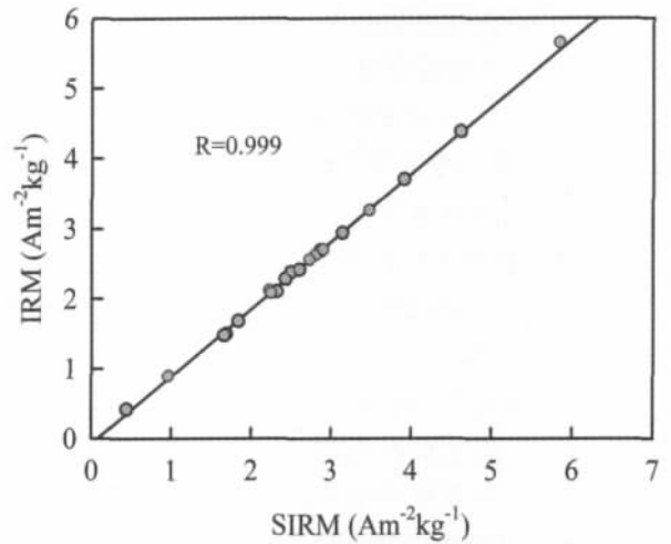
图 2 高砷含水层沉积物样品中饱和等温剩磁与等温剩磁关系图
