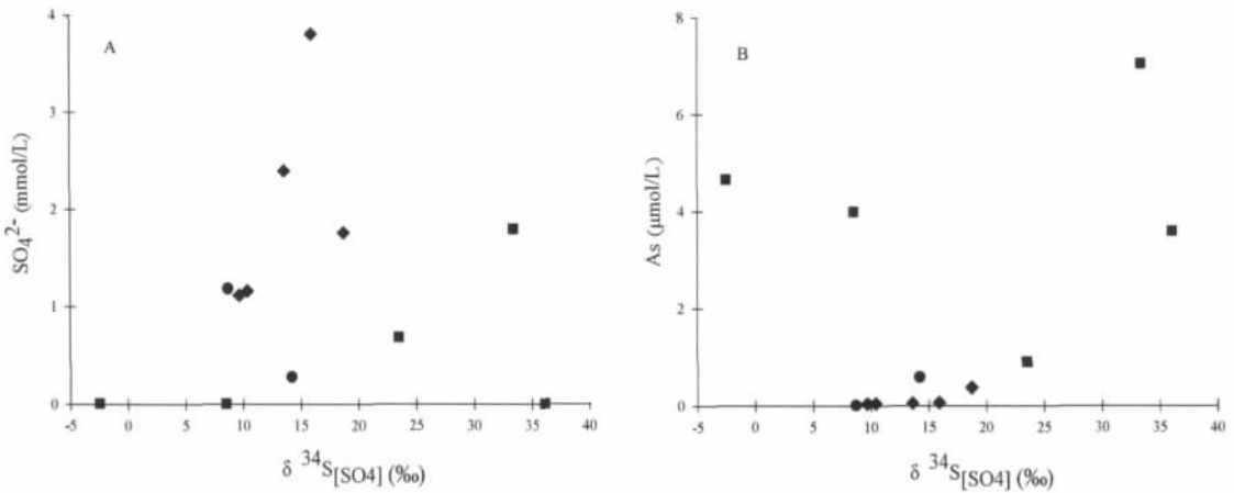
图 6 大同盆地地下水中硫同位素比值与 \text{SO}_4^{2-} 浓度和总砷含量的关系 Fig.6 Content of \text{SO}_4^{2-} and total arsenic versus \delta^{34}\text{S}[\text{SO}_4] in groundwater from Datong basin
