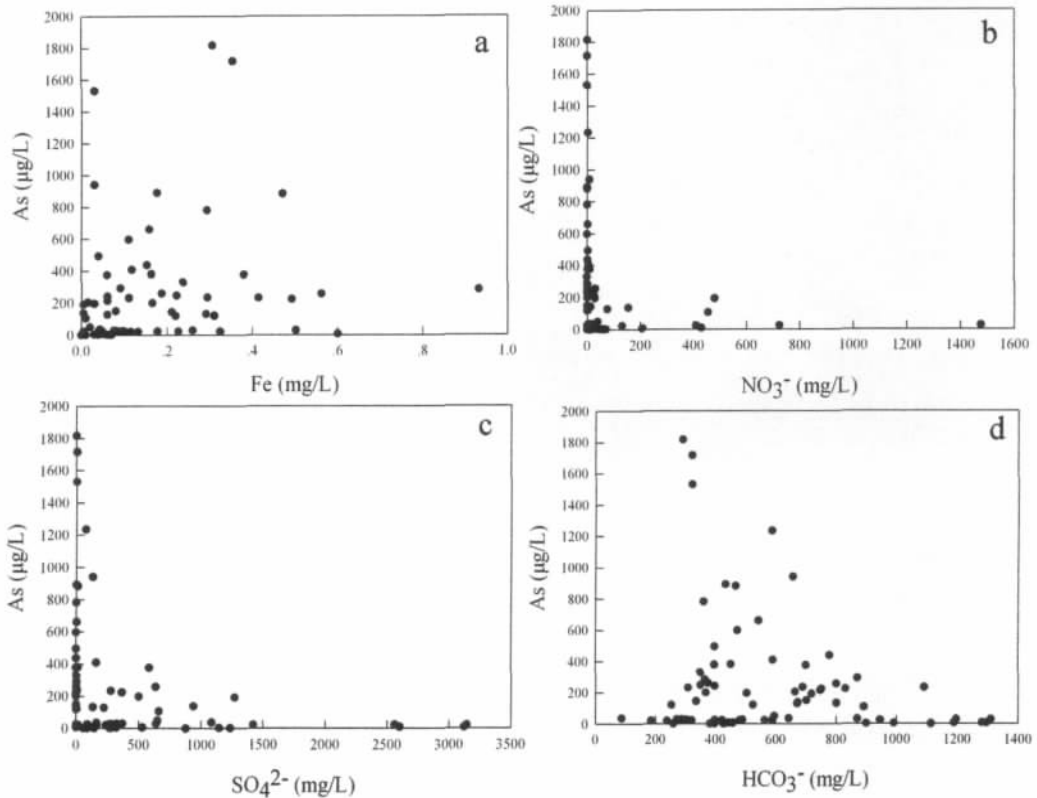
图5 大同盆地高砷地下水中砷与 \text{Fe} 、 \text{NO}_3^- 、 \text{SO}_4^{2-} 、 \text{HCO}_3^- 关系图 Fig.5 The relationship between arsenic and iron (a), nitrate (b), sulfate (c), and bicarbonate (d) in groundwater
