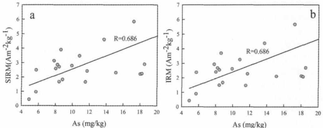
图 3 高砷含水层沉积物中砷含量与环境磁学参数关系图
